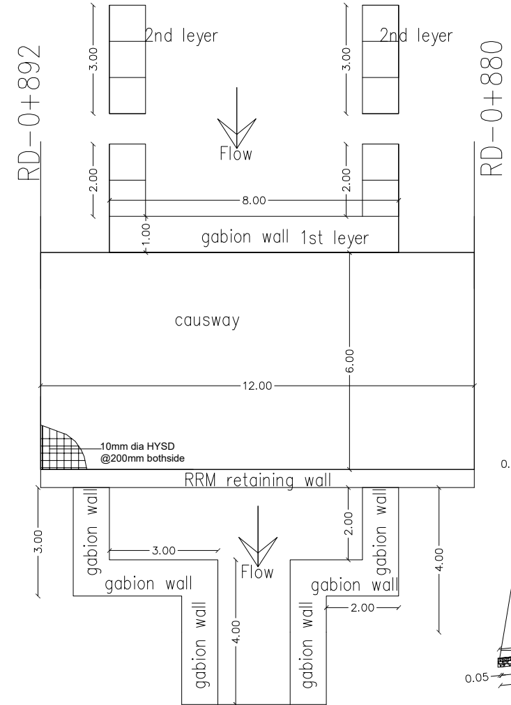
Rd-0+880 to 0+892 PLAN
